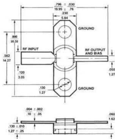
AVANTEK 230 mil BeO FLANGE PACKAGE
