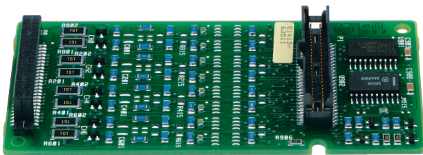
Agilent E1501A
