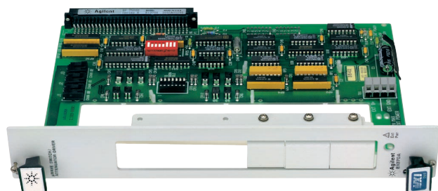
Agilent E1370A
