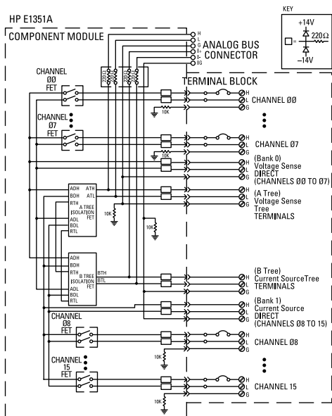
HP E1351A Circuit Diagram
