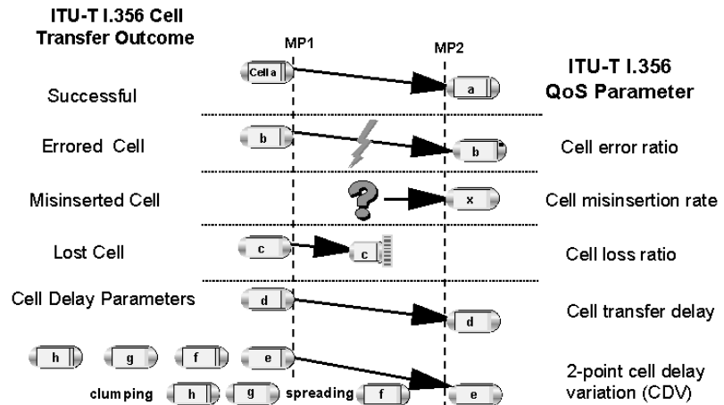
ITU-T I.356 QoS parameters.
