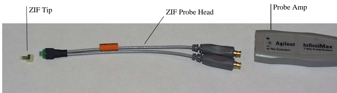
ZIF Probe Head System Components
