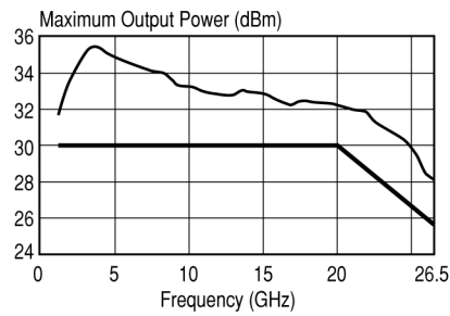
83020A Amplifier
