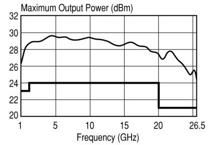
83018A Amplifier
