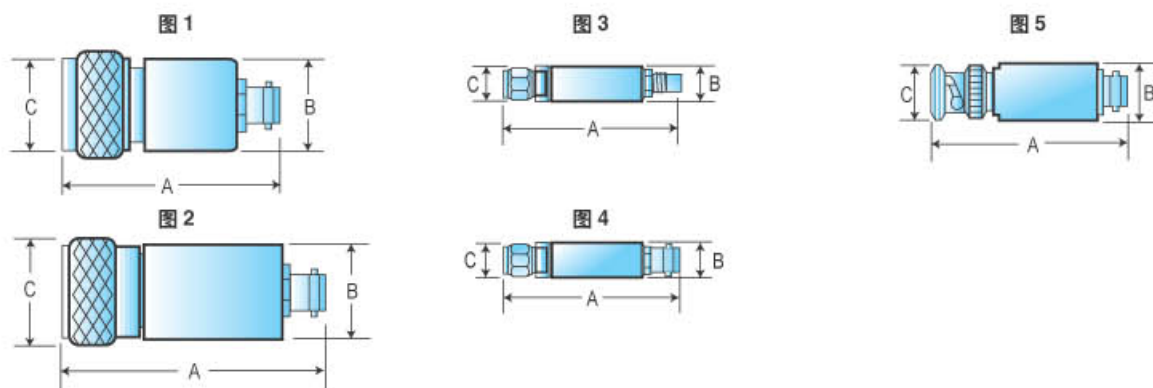
外形图
