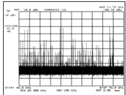
无预选的 50 GHz 至 75 GHz 扫频
