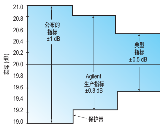
图 2. 保护带例子
