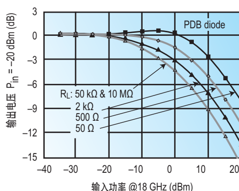
图 8. 典型探测器的平方律响应 (dB)
