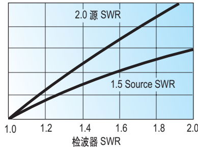
图 5. 检波器和源不匹配造成的失配误差
