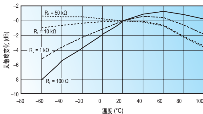
图 3. 典型输出温度响应(Pin < -20 dBm) (肖特基二极管)与温度的关系
