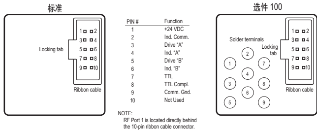
图 6. 驱动连接
