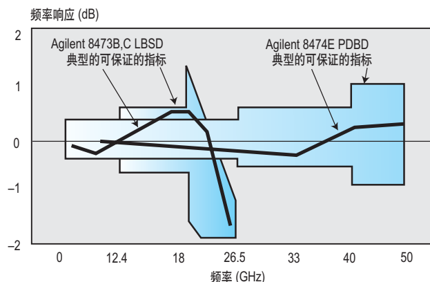
图 1. 检波器频率响应特性
