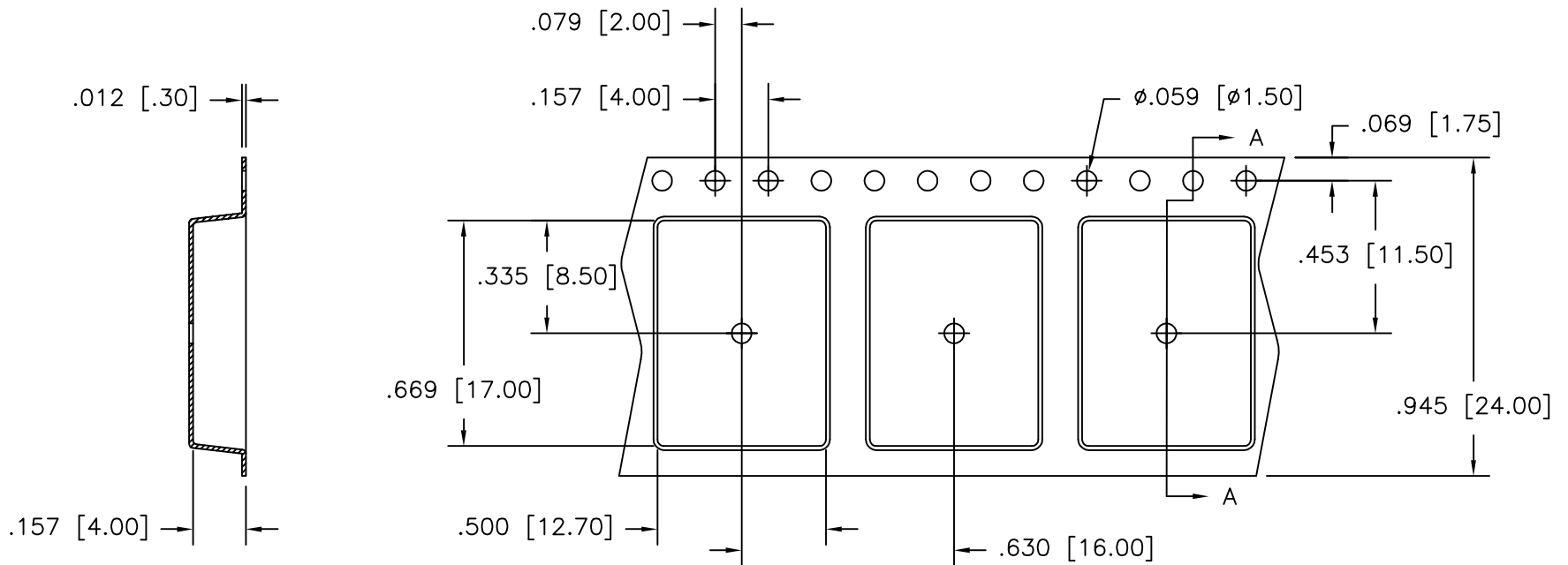
SECTION A-A
