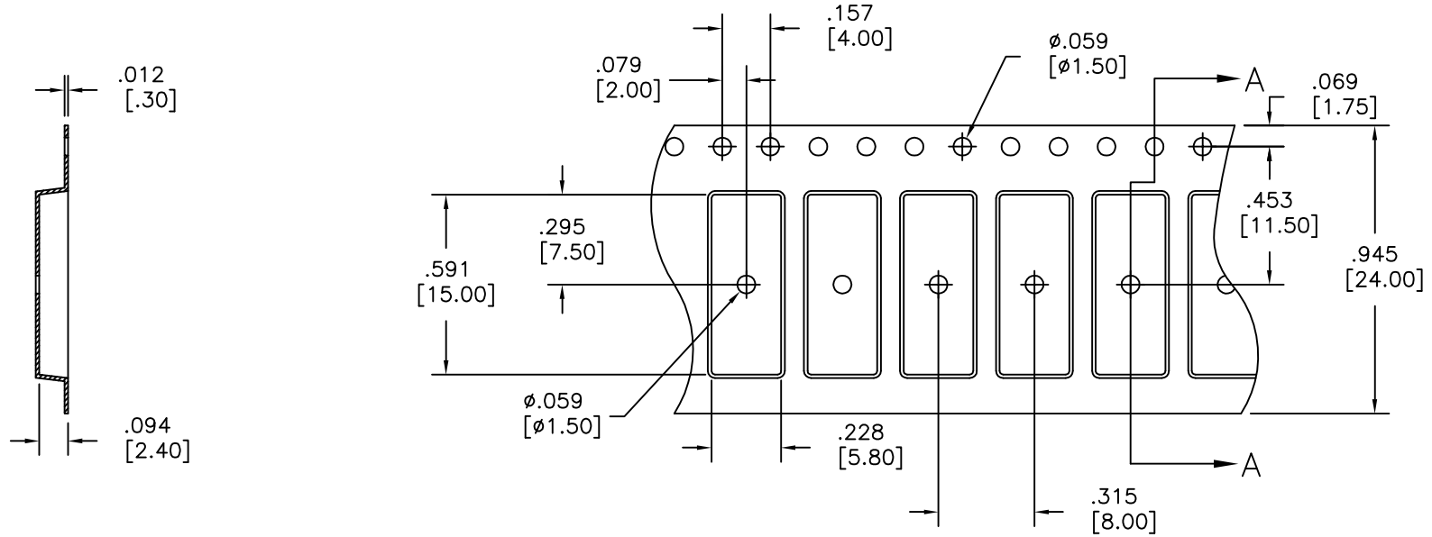
SECTION A-A
