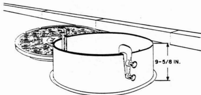
Fig. 1—B or C Manhole Shield
