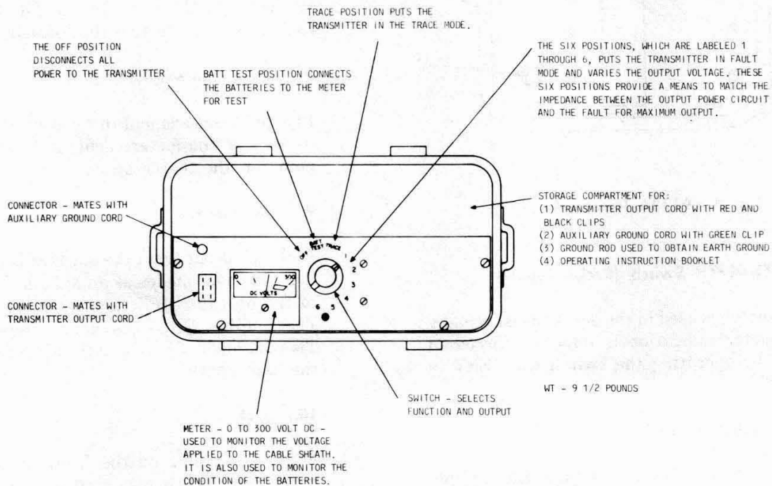
Fig. 3—173A Transmitter
