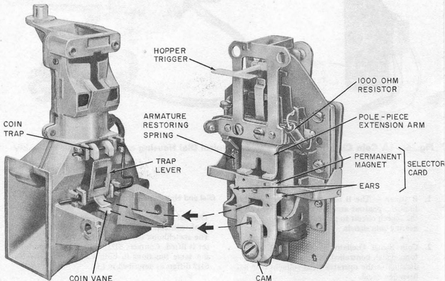
Fig. 8—1AA Coin Relay
