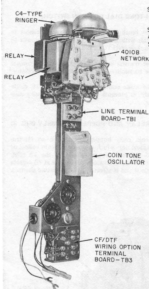
Fig. 6—1A Coin Chassis
