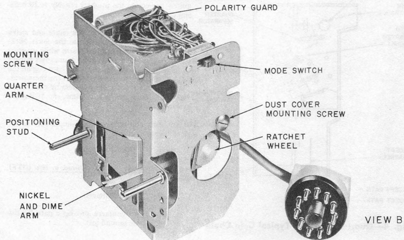
7 Fig. 5—1A Totalizer
