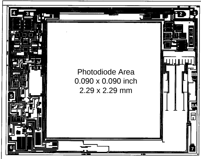
OPT202 DIE TOPOGRAPHY
