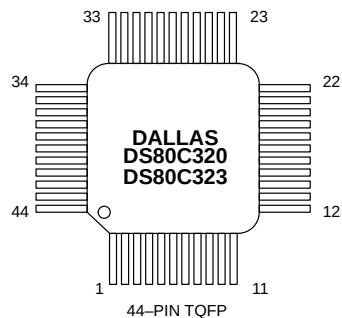
44-PIN TQFP
