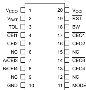
DS1321E 20-PIN TSSOP
