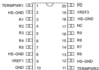
DS21T07E 20-PIN TSSOP (173 MIL)
