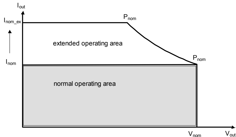
Abbildung 4.1: Arbeitsbereich des Gerätes
