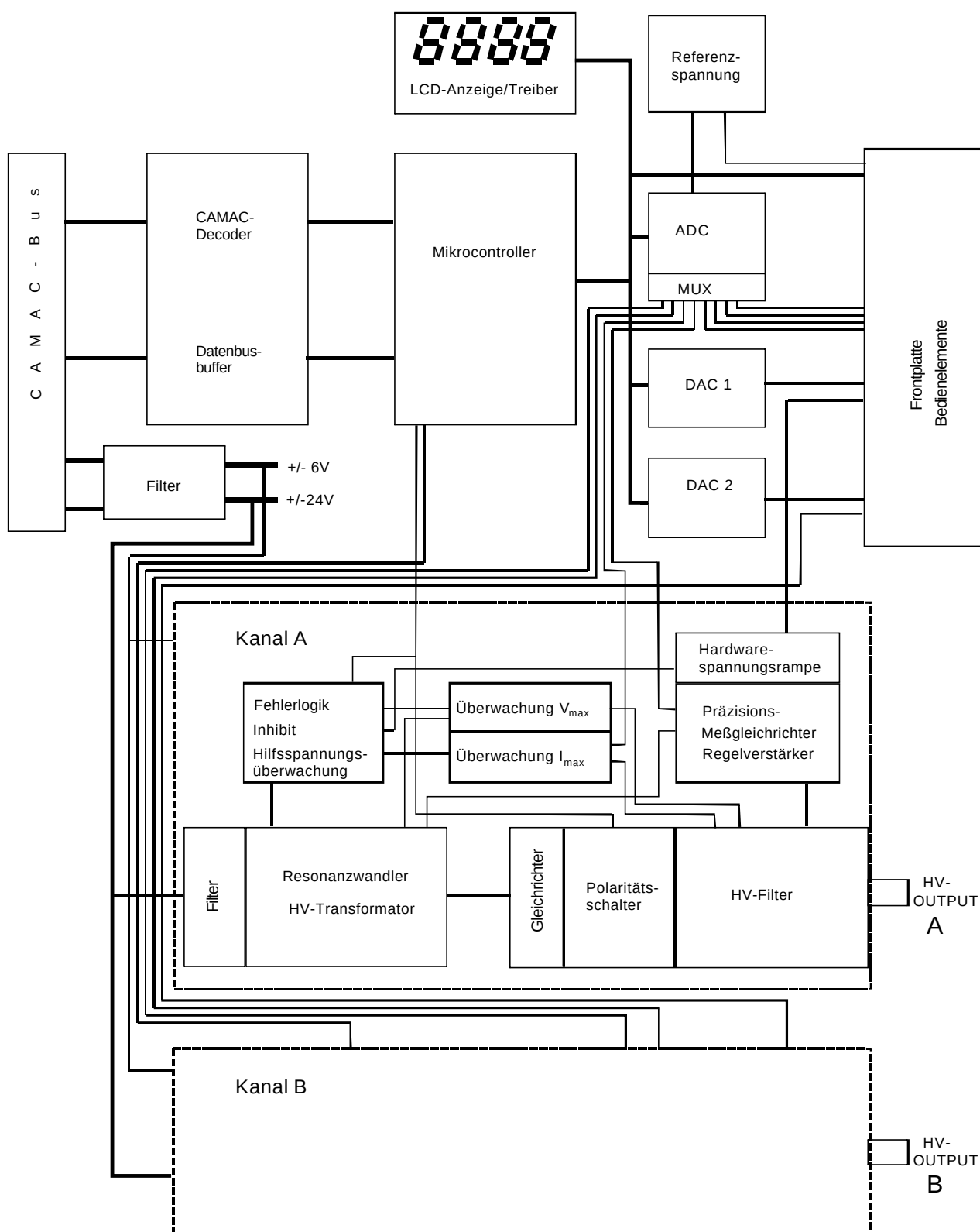
Anhang A: Blockschaltbild CHQ
