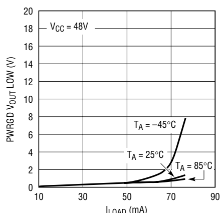
PWRGD V_{\text{OUT}} Low vs I_{\text{LOAD}}
