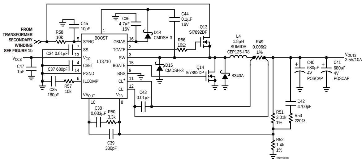
图 1a：36V 至 72V DC 至 3.3V/10A 和 2.5V/10A 双输出隔离电源 (第一部分：后置稳压器电路)
