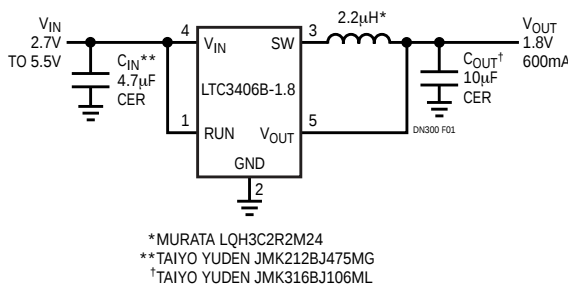
图1：采用全陶瓷电容器的1.8V/600mA降压型稳压器
