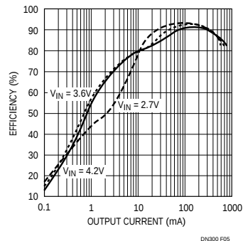
图5: LTC3406B-1.8的效率与负载电流关系
