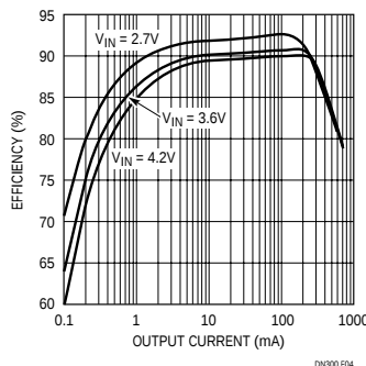
图4: LTC3406-1.8的效率与负载电流关系
