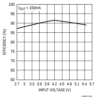
图5：图4所示转换器的效率
