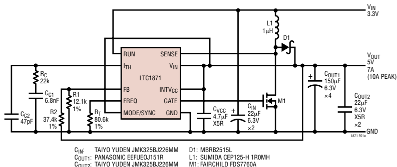
图 1：高效率的 3.3V 输入、5V 输出的升压变换器 (自举型)
