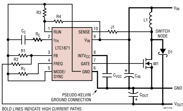
图 15 : LTC1871 升压型变换器的布局图
