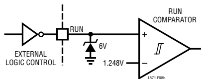
图 8b：采用外部逻辑电路的导通/关断控制
