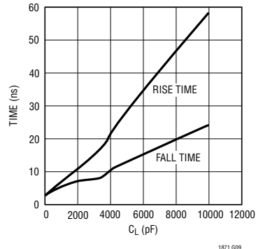
栅极驱动上升和下降 时间与 C_L 的关系
