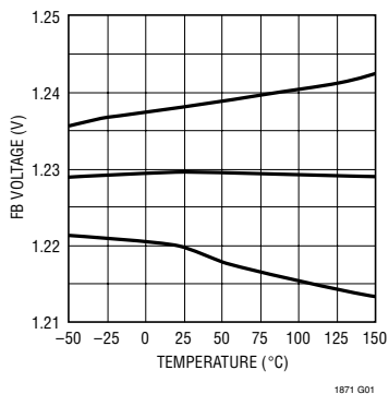
FB 电压与温度的关系
