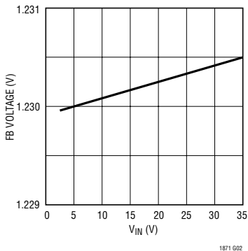
FB 电压调节
