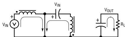
16b : 开关导通期间的电流流动
