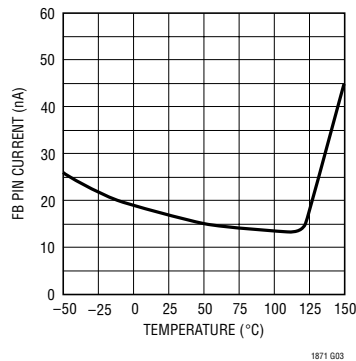
FB 引脚电流与温度的关系
