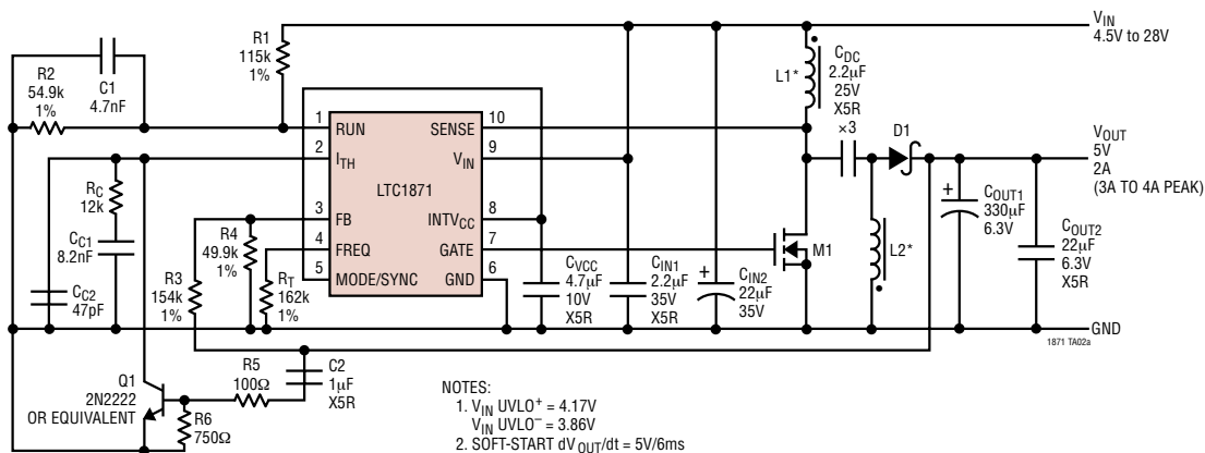
具有欠压关断和软起动功能的 4.5V 至 28V 输入、5V/2A 输出的 SEPIC 型变换器
