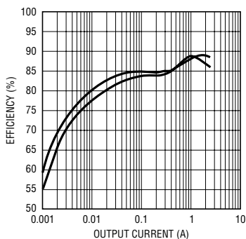
2.5V 和 3.3V 输入时的输出效率
