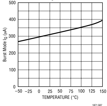
突发方式 I_Q 与温度的关系
