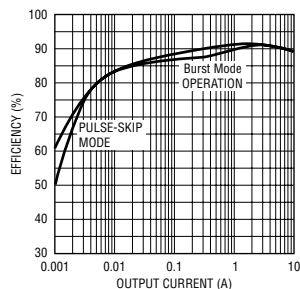
图 1 所示变换器的效率
