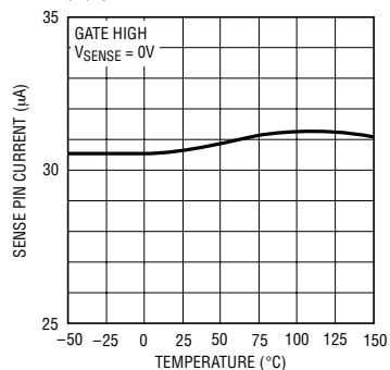
SENSE 引脚电流与温度的关系
