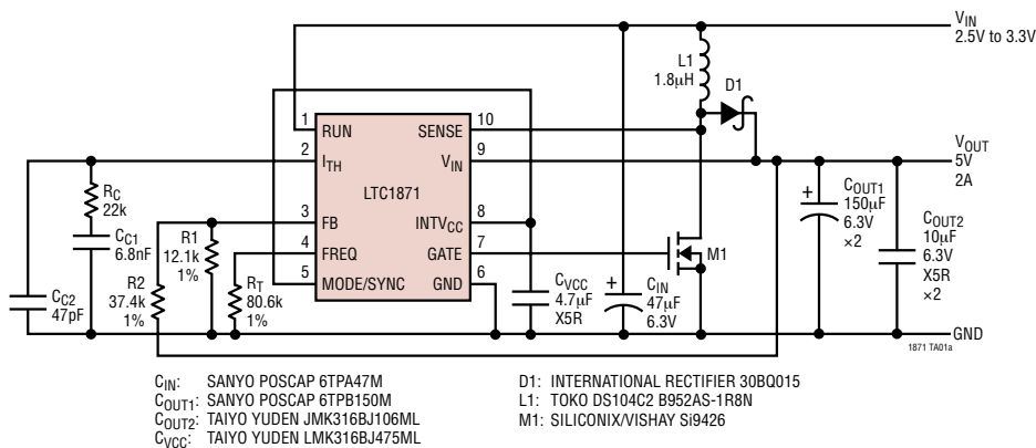
2.5V 至 3.3V 输入、5V/2A 输出的升压型变换器
