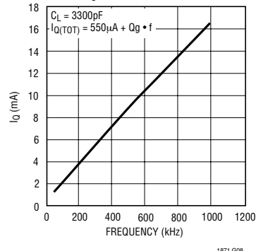
动态 I_Q 与频率的关系
