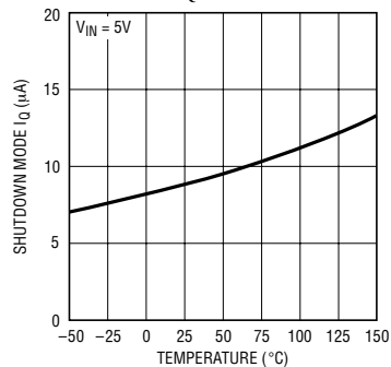
待机模式 I_Q 与温度的关系
