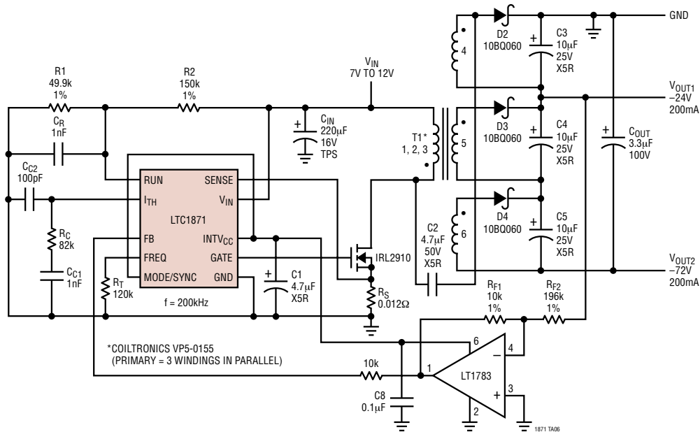
具有欠压关断功能的大功率 SLIC 电源
