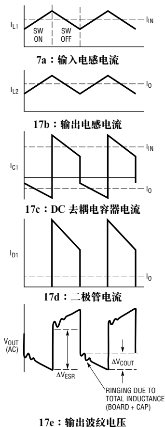
图 17：SEPIC 型变换器开关波形
