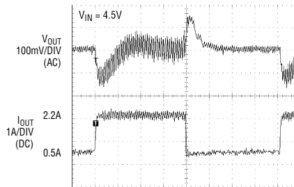
V_{IN} = 4.5V 时的负载阶跃响应
