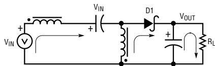
16c : 开关断开期间的电流流动
