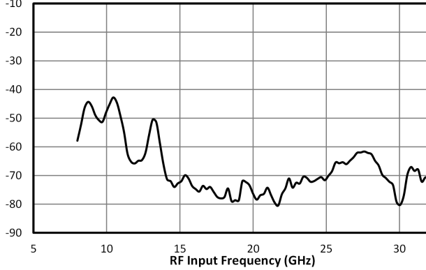
2RF x 2LO Spurious Suppression (dBc) -10 RF dBm input
