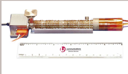
Electron Devices newest millimeter mini TWT the L6083.
