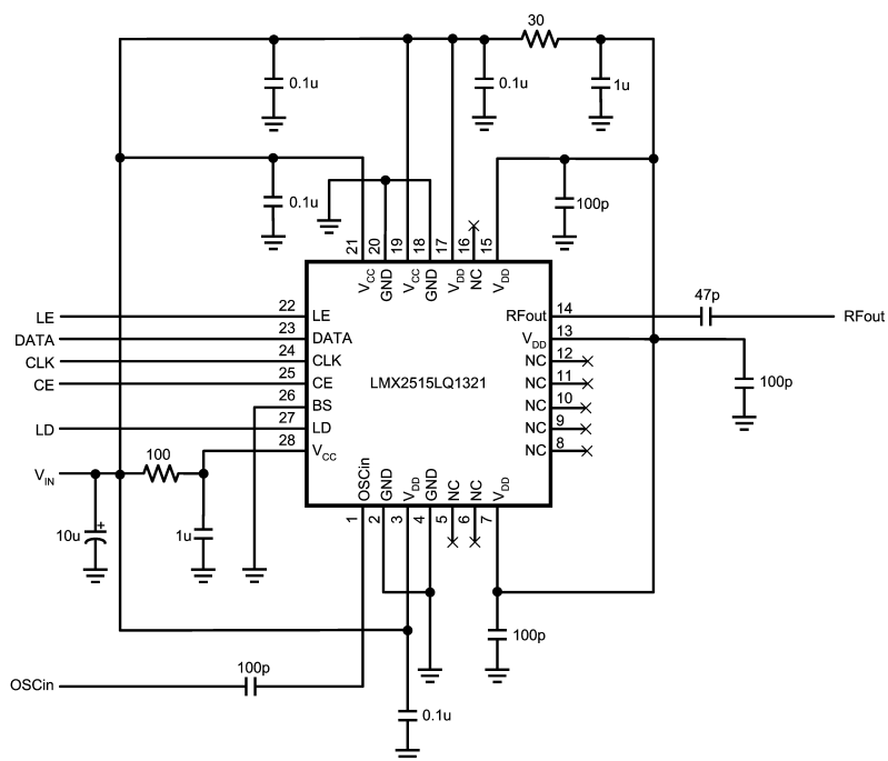
LMX2515LQ1321 Application Circuit
