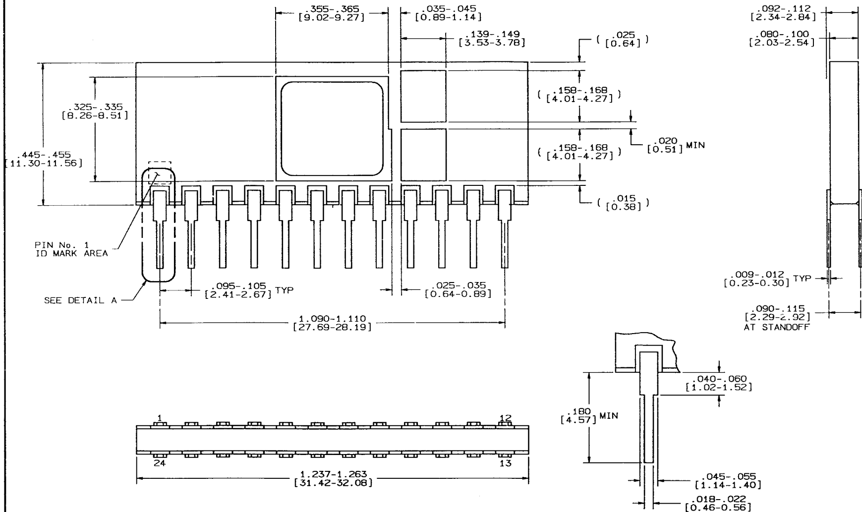
DETAIL A TYP SCALE: 10X
