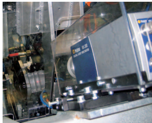
Automatische 100 %-Qualitätskontrolle von Kfz-Komponenten (Foto: P. Marpe, TRW Automotive)
