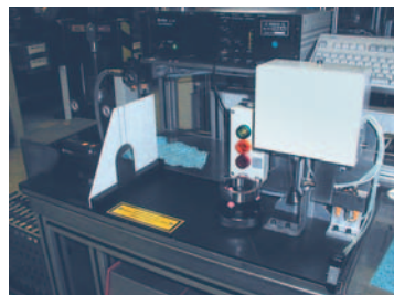
Testaufbau für die akustische Qualitätskontrolle mit einem Industrial Vibration Sensor
