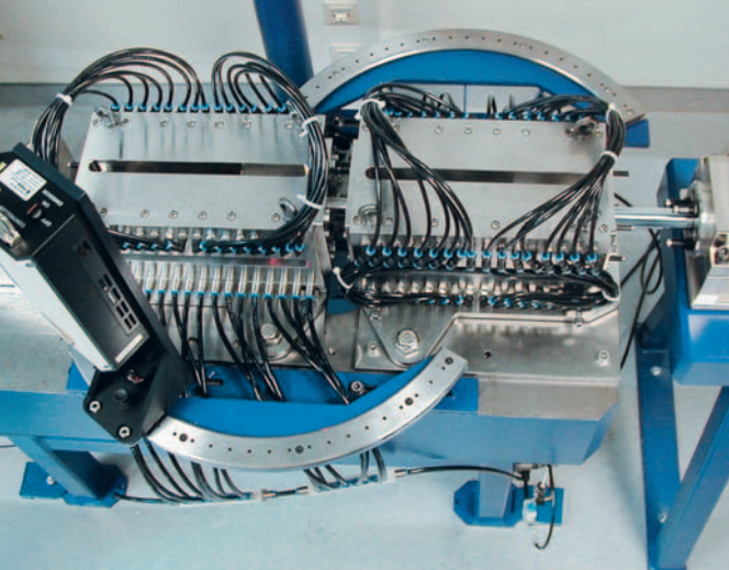
Kalibration von Impulskräften mit einem Laserinterferometer
