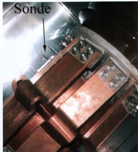
Bild 6. Faseroptische Temperaturmessung an der Stromdurchführung eines Transformators
