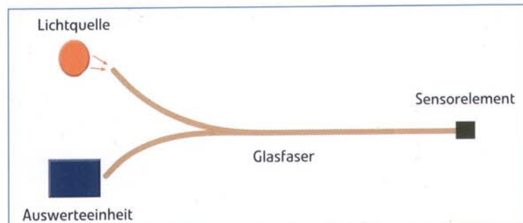
Bild 1. Schema extrinsischer faseroptischer Sensoren
