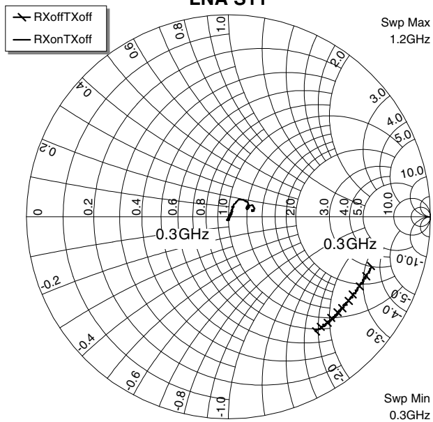
LNA S11
